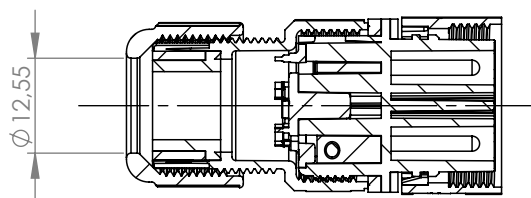
SEZIONE A-A
