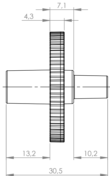
DETTAGLIO B SCALA 3 : 1
