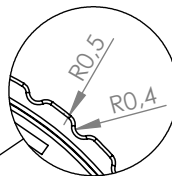
DETTAGLIO B SCALA 3 : 1
