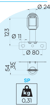
SP Spinotto con attacco a parete
