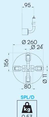
SPL/D Spinotto orientabile dritto
