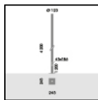
S.2846 PALE CILINDRICO H 4,2m f.t., Ø120mm FLANGIATO
