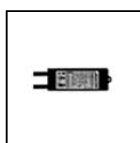
S.2448 ALIMENTATORE ON-OFF 31W 230Vac/48Vdc IP67 Alimentatore per led monocolori 31W 230Vac/48Vdc Il numero massimo degli apparecchi collegabili dipende dalla somma delle singole potenze. IP67 CLASSE II SELV Dimensioni 120x38x25mm SI CONSIGLIA L'UTILIZZO DELLO SCARICATORE DI SOVRATENSIONE S.2499 PER OGNI ALIMENTATORE ELETTRONICO CHE DEVE ESSERE INSTALLATO A MAX 10m DI DISTANZA DA QUEST'ULTIMO.
