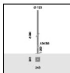
S.2848 PALO CILINDRICO H 6,0m f.t., Ø120mm FLANGIATO
