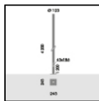
S.2846 PALO CILINDRICO H 4,2m f.t., Ø120mm FLANGIATO
