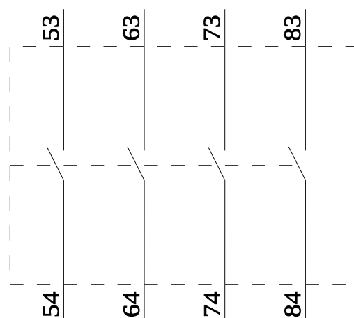
3RH2
