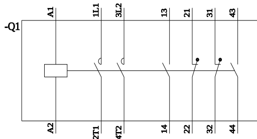
3TY7684-0Qxx
