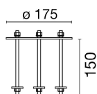
Piastra tirafondi acciaio zincato verniciato - Adatta per base da pavimento
