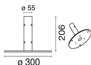
Base palo da pavimento 60mm - Adatto per palo H 3m
