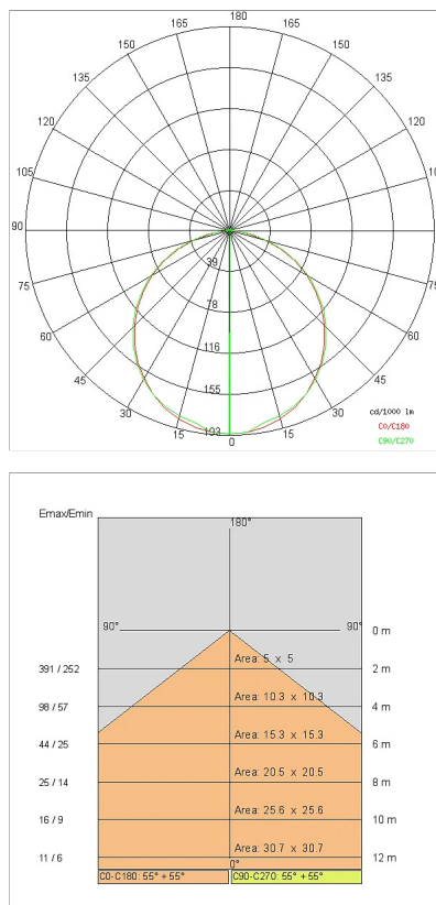
CURVE FOTOMETRICHE
