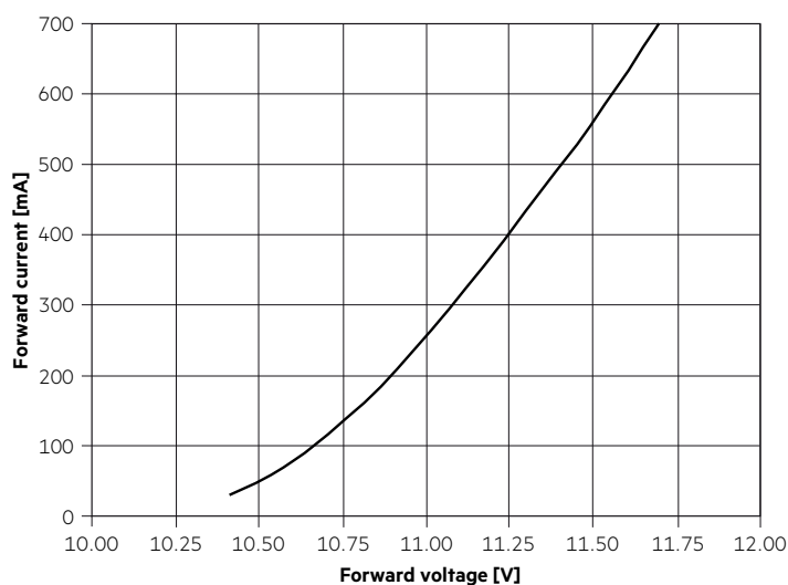
LLE 24x140mm 650lm 8xx HV ADV6
