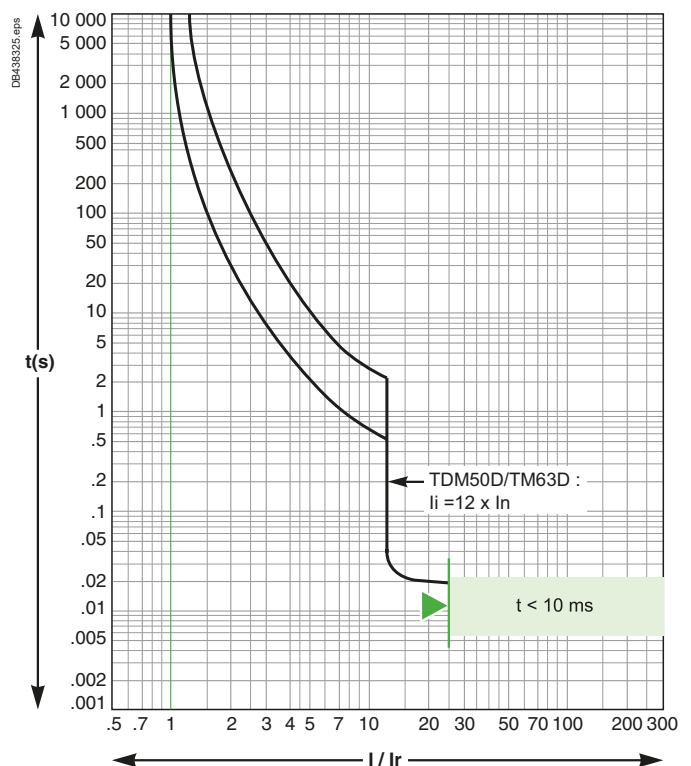
TM50D/TM63D
