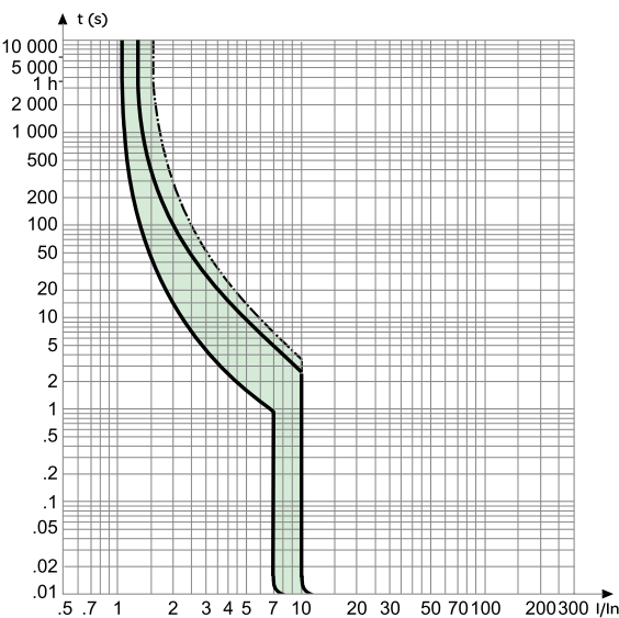
C 曲线
