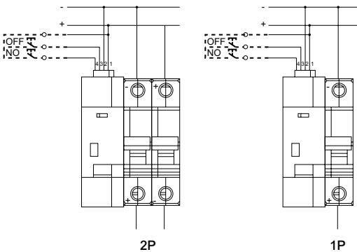
接线图
