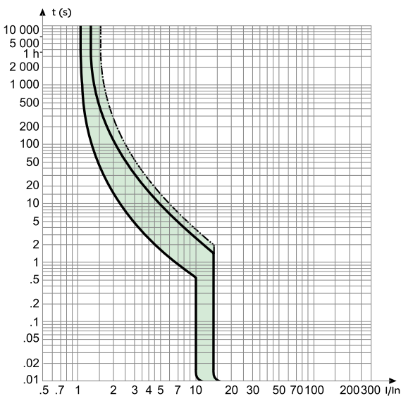
D 曲线
