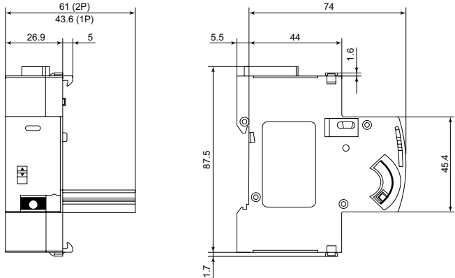
尺寸(mm)
