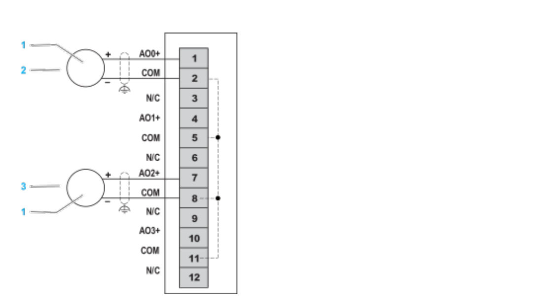
1: Attuatore 2: connessione a 2 fili per uscita di tensione 3: connessione a 2 fili per uscita di corrente
