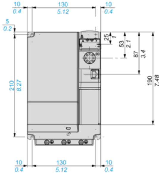
Vista destra e anteriore con piastra EMC
