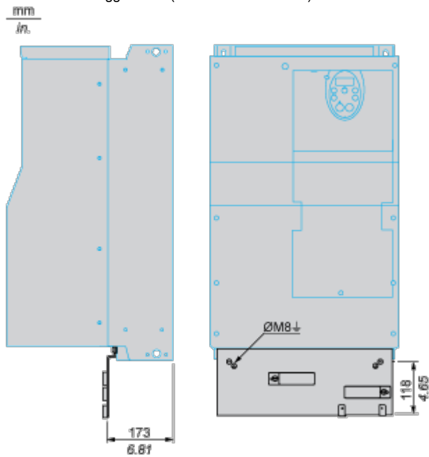
Piastra di montaggio EMC (fornita con il variatore)
