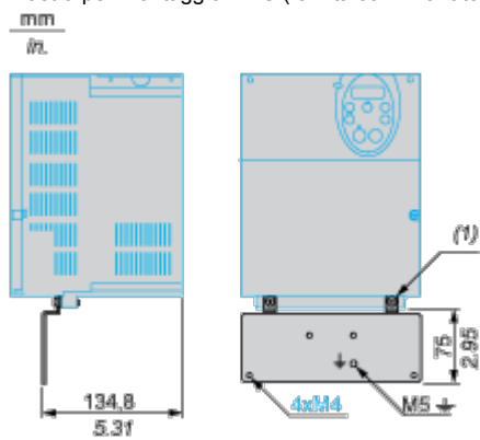
Piastra per montaggio EMC (fornita con il variatore)
