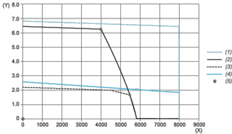
Curve di coppia/velocità con alimentazione trifase 480 V
