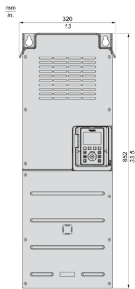
Azionamenti senza coperchio IP21 Viste destra e anteriore
