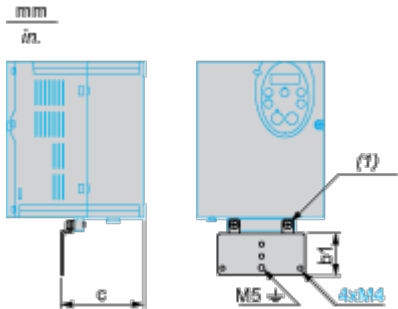
(1) 2 viti M5
