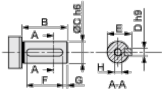
DIN 6885 A
