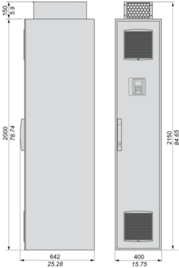
Viste destra e anteriore
