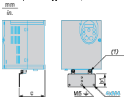
(1) 2 viti M5
