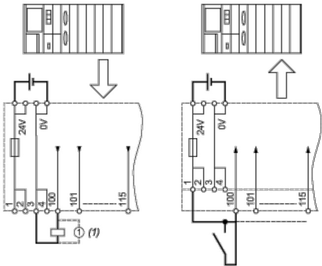
(1) Carico induttivo
