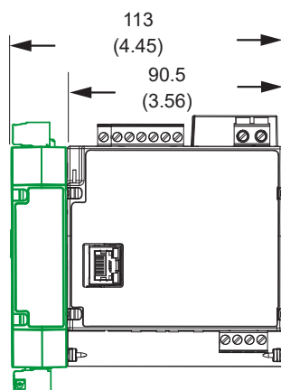
ION7403 / ION7413
