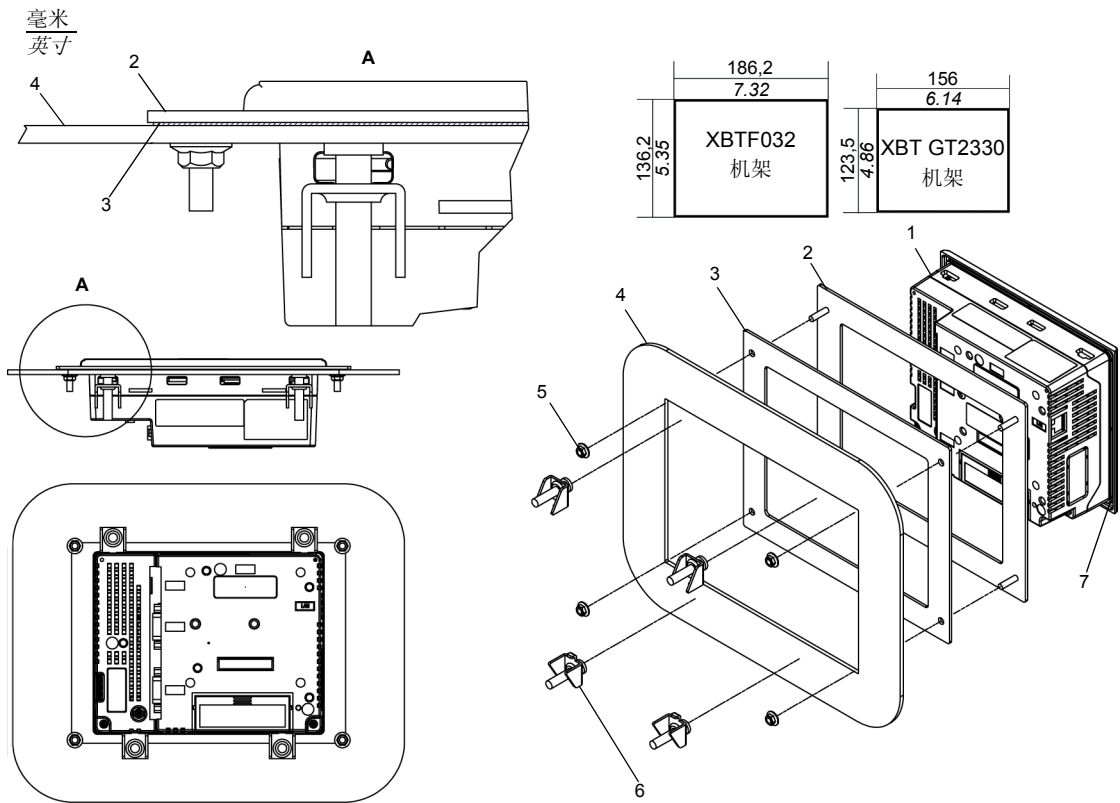
示意图中的主要组件及配件。
