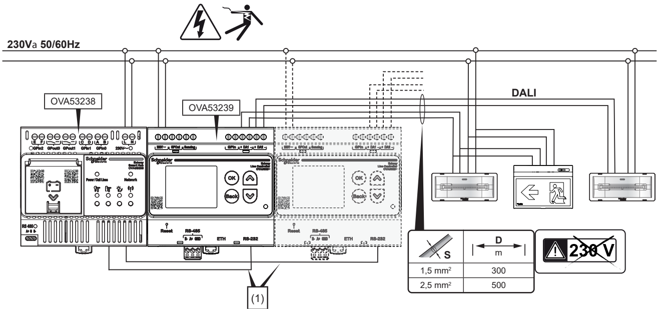
(1) Connettere la Schermatura del cavo ad un solo capo della linea.
