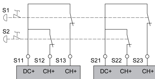
Cablaggio degli ingressi per le protezioni
