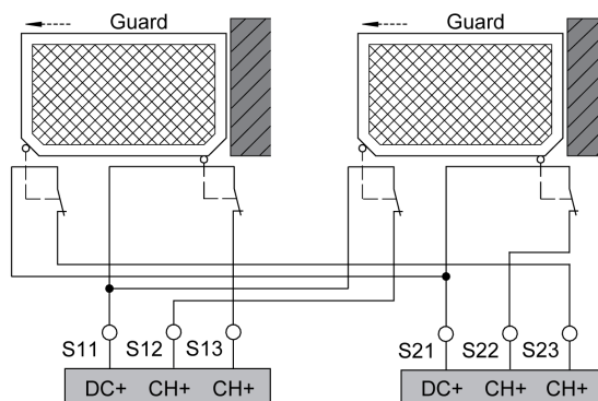
Cablaggio degli ingressi per le protezioni
