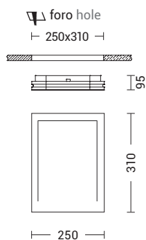
TASCA002MT cassaforma per muratura casting box
