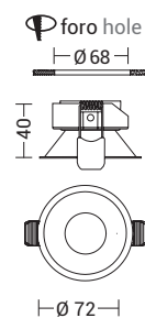
RAS003B ghiera con cornice arretrata backward ring
