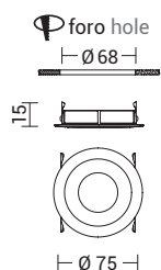
RAS002B ghiera con cornice shelf shelf ring
