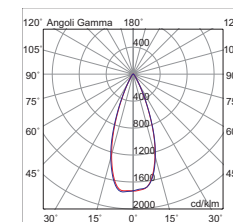
diagramma polare 13W 13W polar diagram
