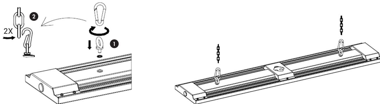
FIG. 2 - KIT SOSPENSIONE SUSPENSION KIT
