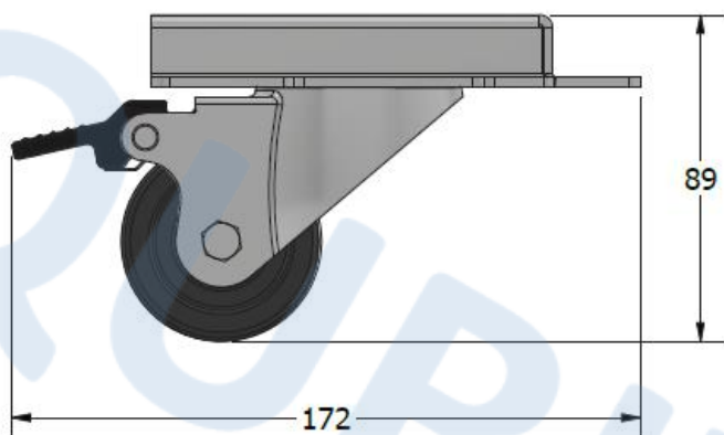
Vista frontale
