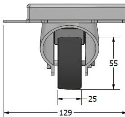
Vista laterale
