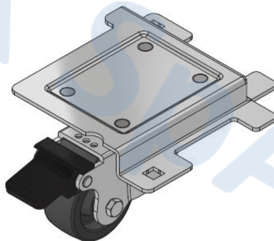
Vista isometrica
