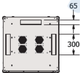
Vista dall'alto per armadi con L=800
