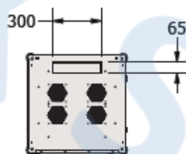
Vista dall'alto per armadi con L=600
