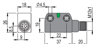
Sensore ST G••••M• con connettore M12
