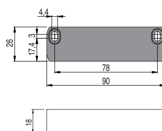
Azionatore SM E•T
