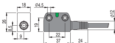
Sensore ST G••••N• con cavo
