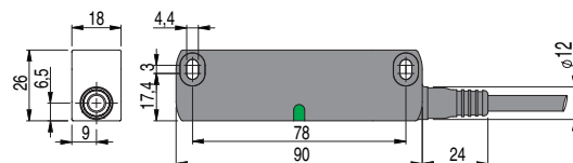
Sensore ST H••••N• con cavo
