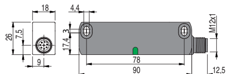
Sensore ST H••••M• con connettore M12
