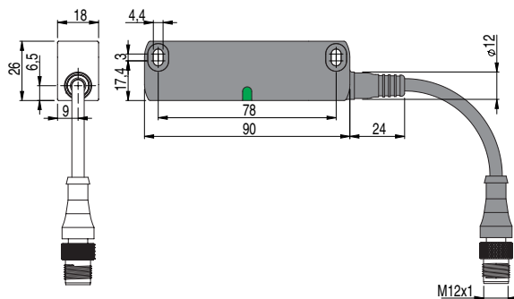
Azionatore SM H•T
