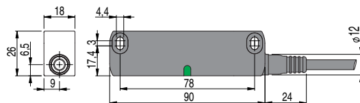
Sensore ST H••••M• con connettore M12
