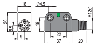
Sensore ST G••••M0.2 con cavo e connettore M12
