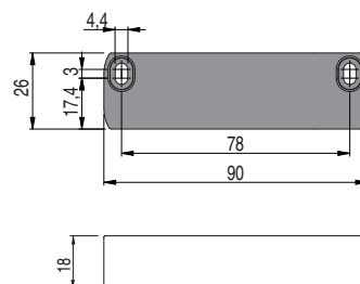
Azionatore SM E•T
