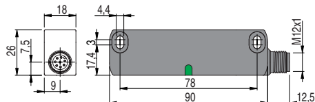
Sensore ST H••••M0.2 con cavo e connettore M12
