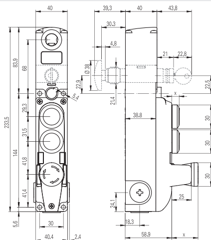
Interruttore NG 2D●●●●●● con dispositivi di comando integrati
