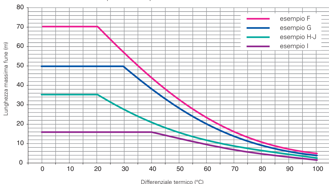
Campate massime per interruttori con testa trasversale
