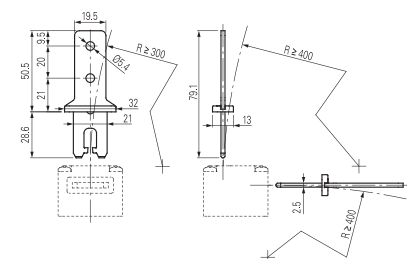
Azionatore VF KEYF20
