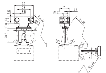
Azionatore VF KEYF28
