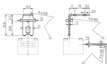
Azionatore VF KEYF28
