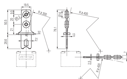
Azionatore VF KEYF22
