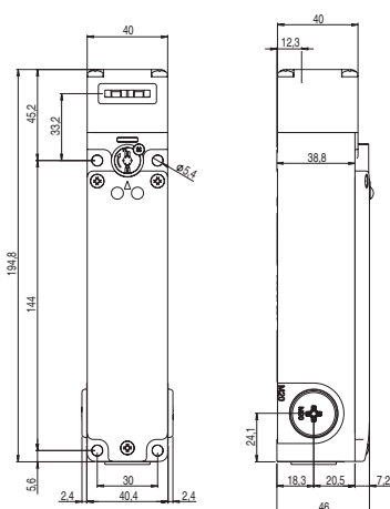
Interruttore FG 6•D6D•• Principio di funzionamento D con sblocco ausiliario a serratura e pulsante di sblocco antipanico
