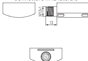
Connettore M12 laterale
