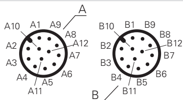
Doppio connettore M12 a 12 poli
