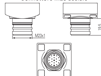
Connettore M23 assiale
