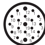
Connettore M23 a 19 poli
