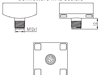
Connettore M12 assiale
