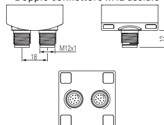
Doppio connettore M12 assiale
