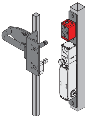
Dispositivo di lock out aperto. Interruttore di sicurezza accessibile.
