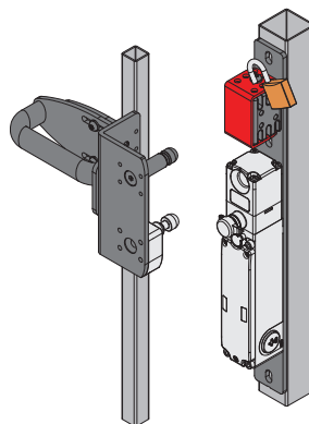
Dispositivo di lock out chiuso. Inserimento lucchetto.
