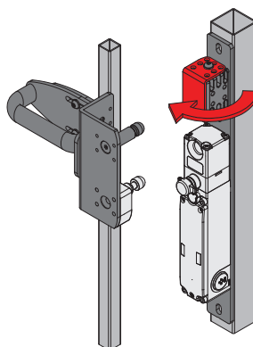
Chiusura dispositivo di lock out.
