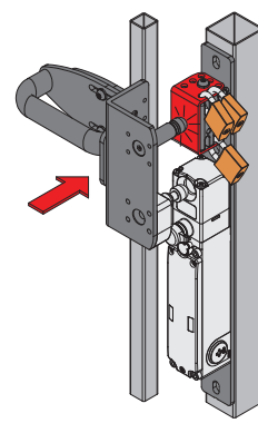
Dispositivo di lock out bloccato. Lucchetto bloccato. Interruttore di sicurezza non accessibile.
