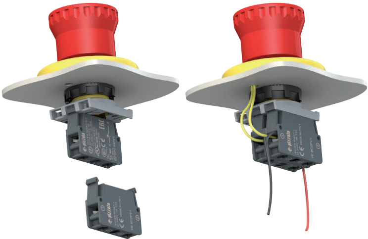
Cablaggio con blocco di connessione
