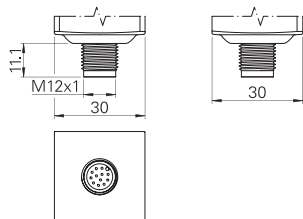
Connettore M12 assiale
