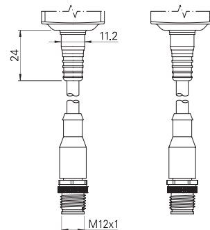
Con cavo lunghezza 0,2 m e connettore M12 assiale
