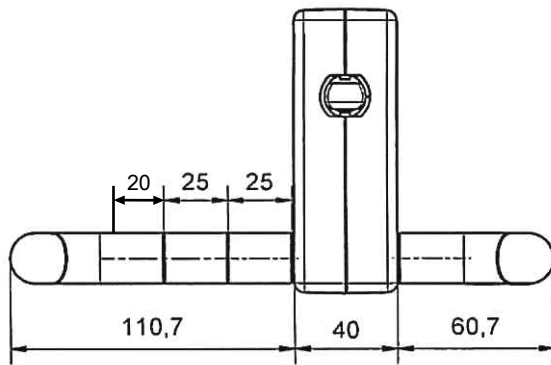
Abb.: Seitenansicht des Betätigers mit zwei Verlängerungen (Bestell-Nr. 6O000009)
