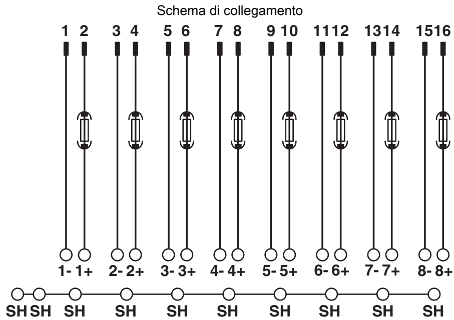
Schema di collegamento UM-DELTA V/D/SI/BFI/TP
