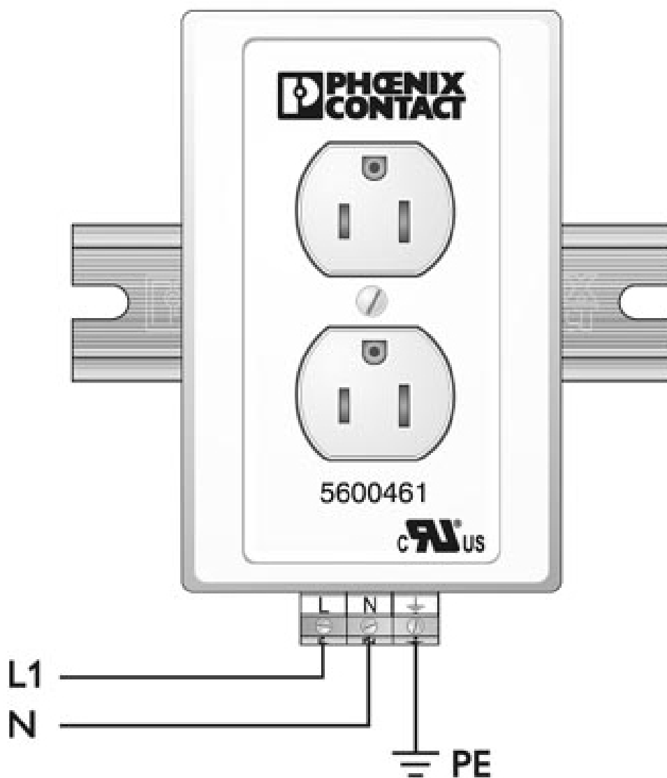
Disegno collegamento
