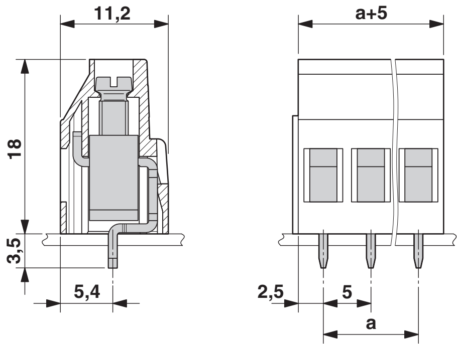
Disegno quotato
