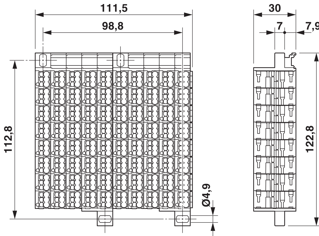
Disegno quotato
