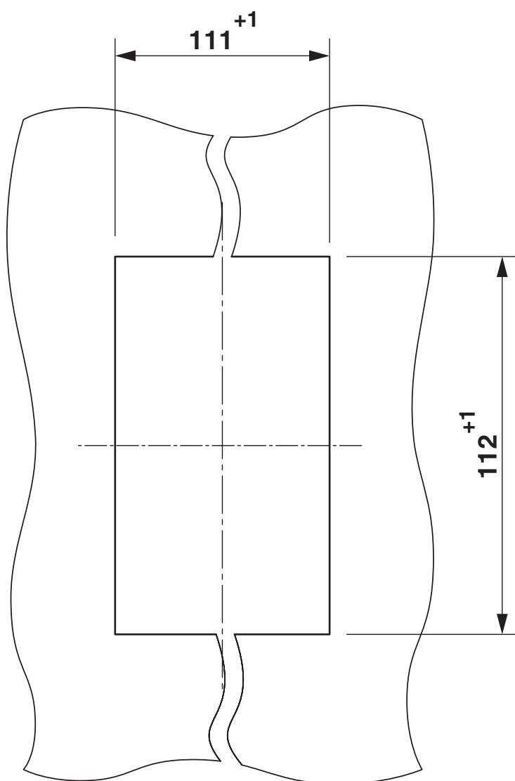
Disegno quotato
